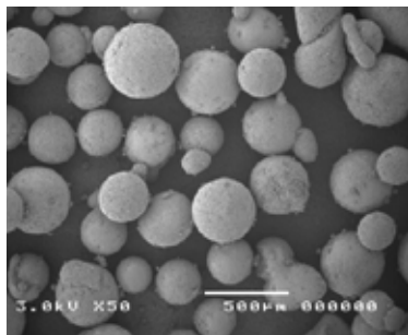
Granuler av ett kompositmaterial framtagna via frysgranulering.
