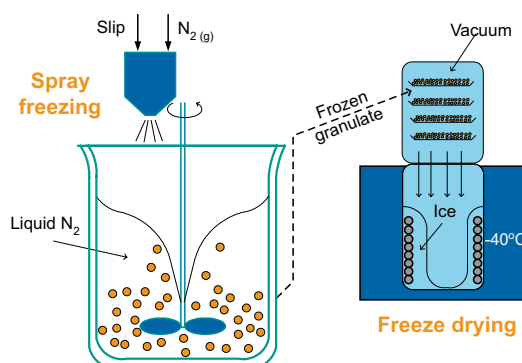
Illustration av processen vid frysgranulering.
